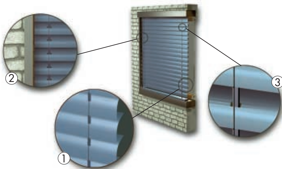
Abb. 4.1.1-2: Wichtige Punkte für die Auswahl einer Außenjalousie
