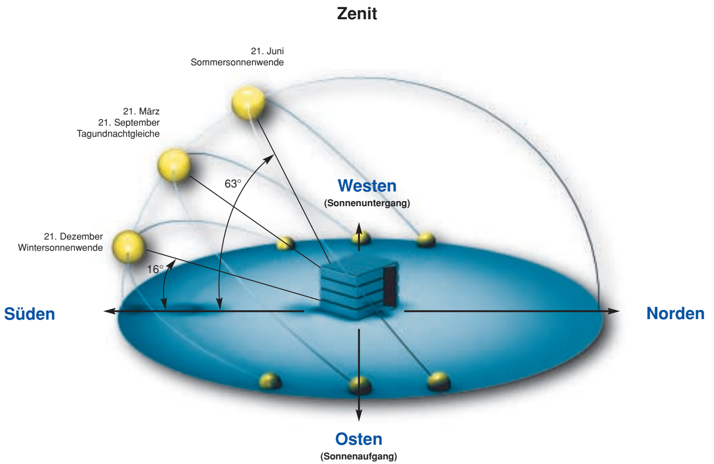
Abb. 1-2: Verlauf der Sonne für Mitteldeutschland
