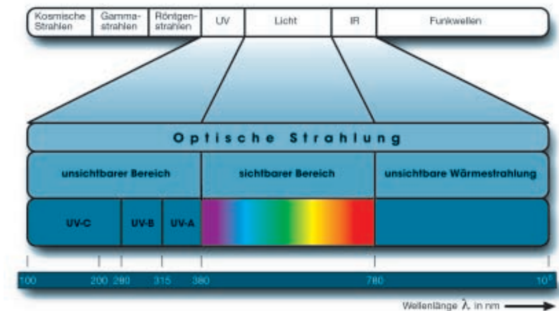
Abb. 1-1: Spektrum der elektromagnetischen Strahlung
